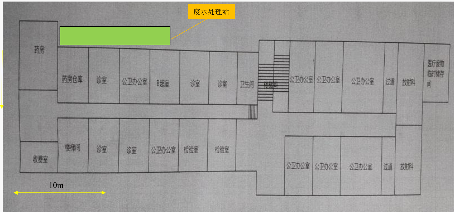
附图4-1 一层平面布置图
