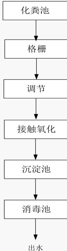
图3-3 污水处理工艺图
